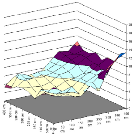
Magnetische Flussdichten 105 cm oberhalb der mit Stahl armierten Bodenplatte
