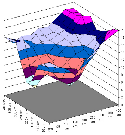
Magnetische Flussdichten 55 cm oberhalb der mit Stahl armierten Bodenplatte
